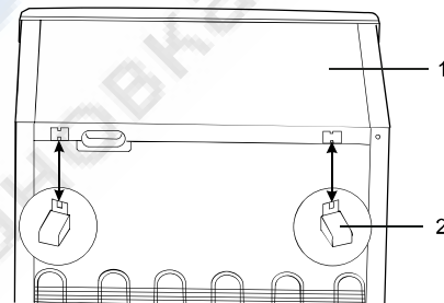
Рисунок Б.2 - Схема крепления упорів до кришки Рисунок Б.2 - Схема крепления упоров к крышке Şəkil B.2 - Dayaqların qarağa bərkidilmə sxemi ნაპაბო Б.2 - სახურავზე საყრდენების დამაგრების სქემა Б.2-сурет - Тіреуішті қақпаққа бекіту схемасы Figura B.2 – Schema fixării de sarac a opritorului B.2-rasm: Tirgakların ustki qismga oʻrnatish chizmasi.
